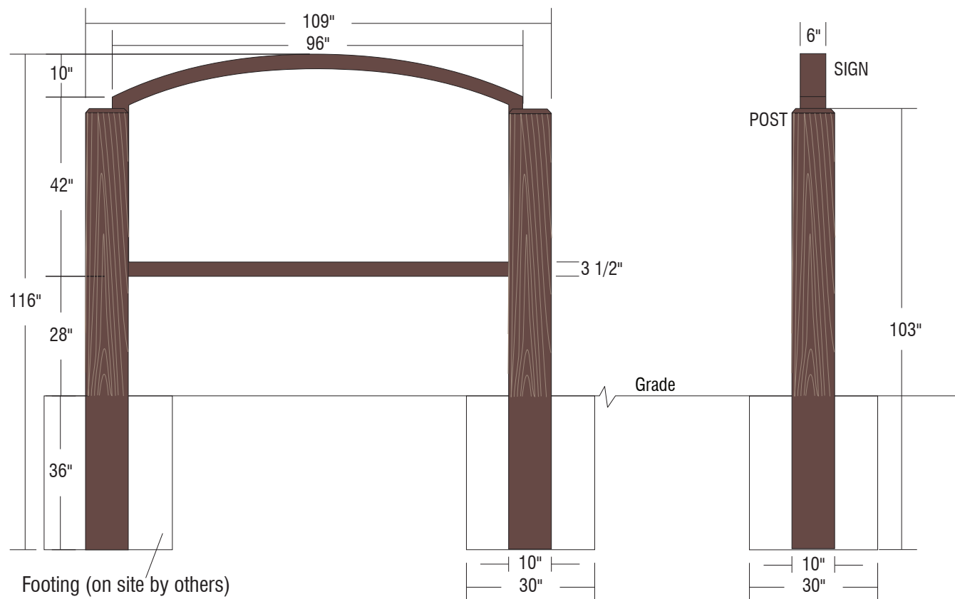
ELEVATION
